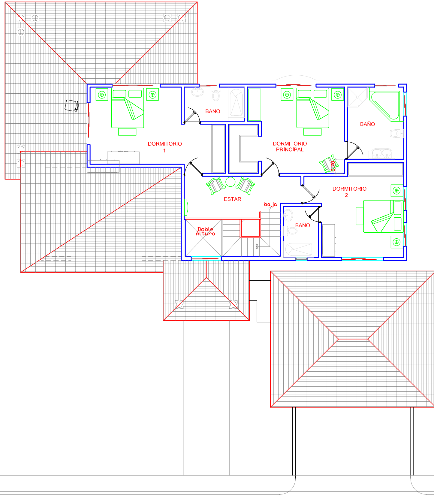
Planta Amueblada SEGUNDO NIVEL AREA= 118.50M 2
