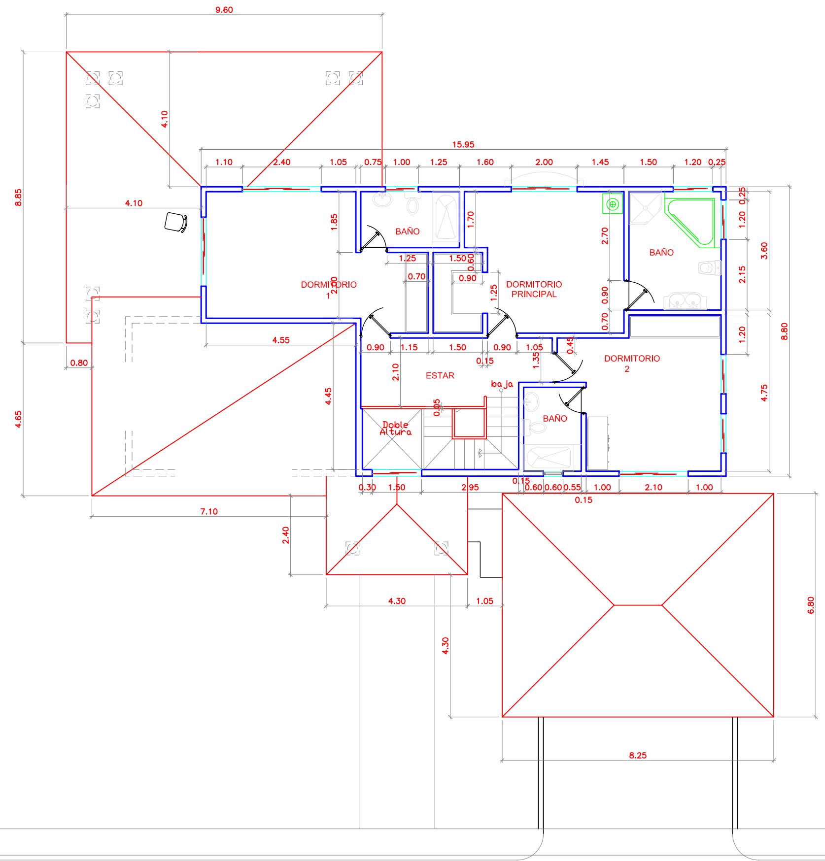
Planta Dimensionada SEGUNDO NIVEL AREA= 118.50M 2
