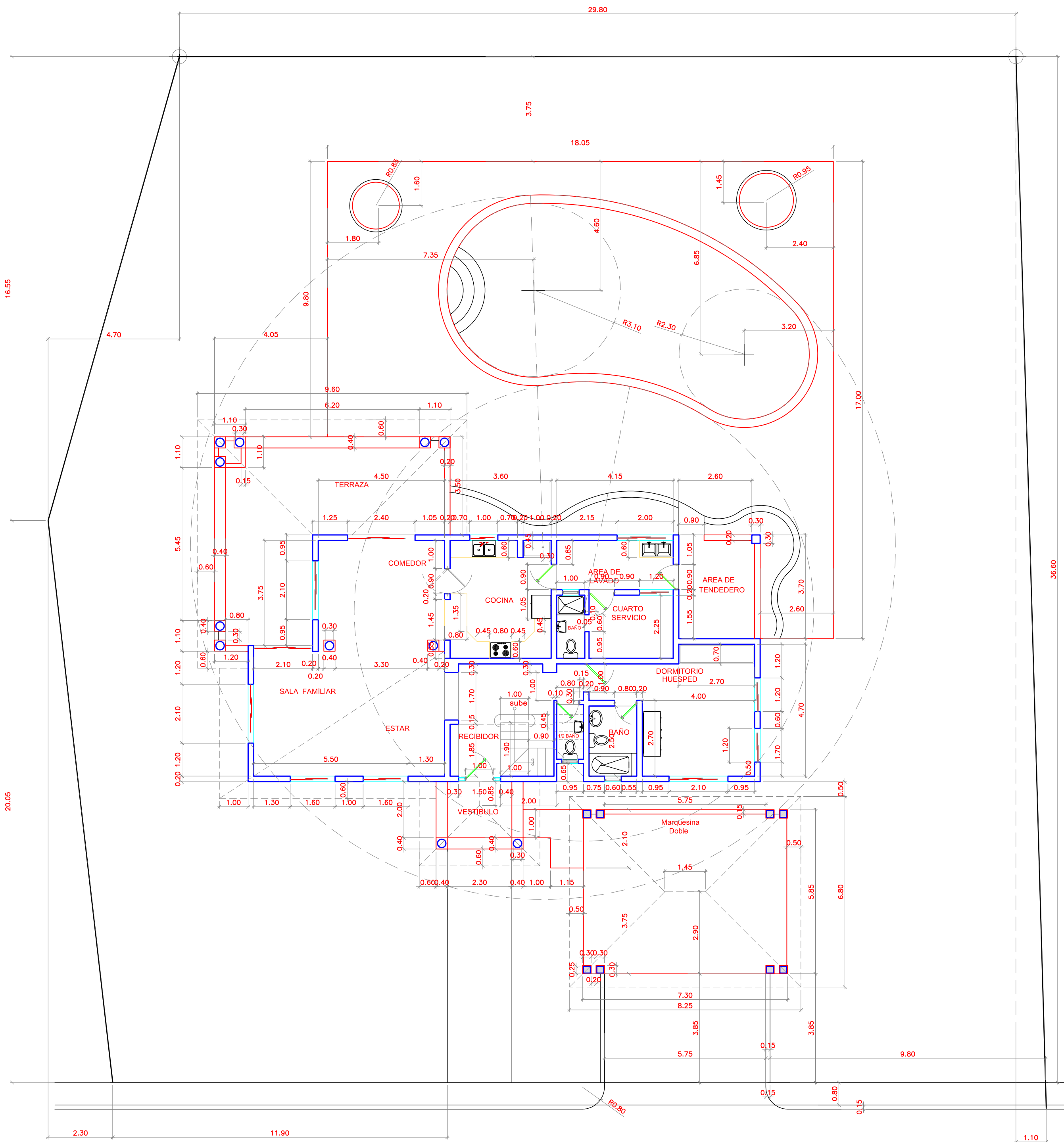
Planta Dimensionada PRIMER NIVEL AREA=245.10M2
